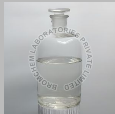
Methoxyacetyl Chloride
